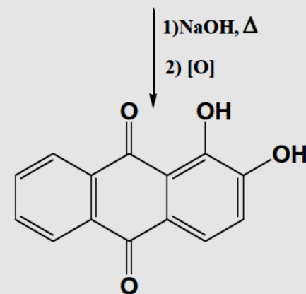
Alizarine
