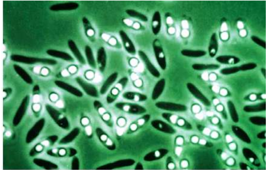
(d) Desulfotomaculum : phase-contrast microscopy
