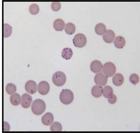
Fig: Mycoplasma
