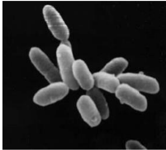
Fig: Archaeobacteria
