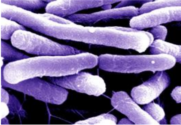
Fig: E.coli
