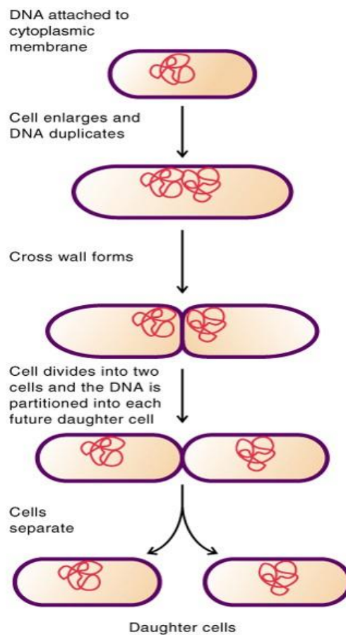
Fig: Binary
