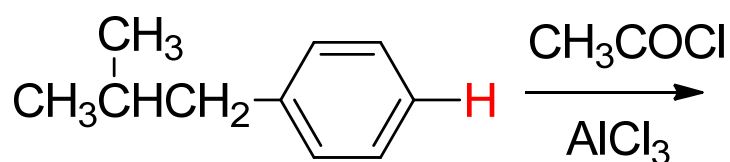
iso-butylbenzene
